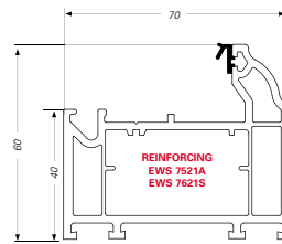
OVOLO MAIN FRAME - EWS 7721
