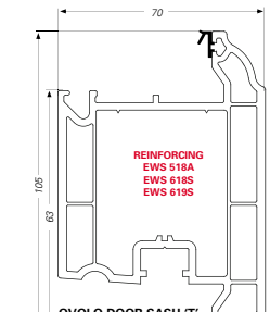
OVOLO DOOR SASH 'T' - EWS 7719
