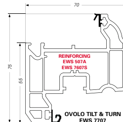
OVOLO TILT & TURN - EWS 7707
