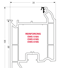
OVOLO DOOR SASH 'Z' - EWS 7718
